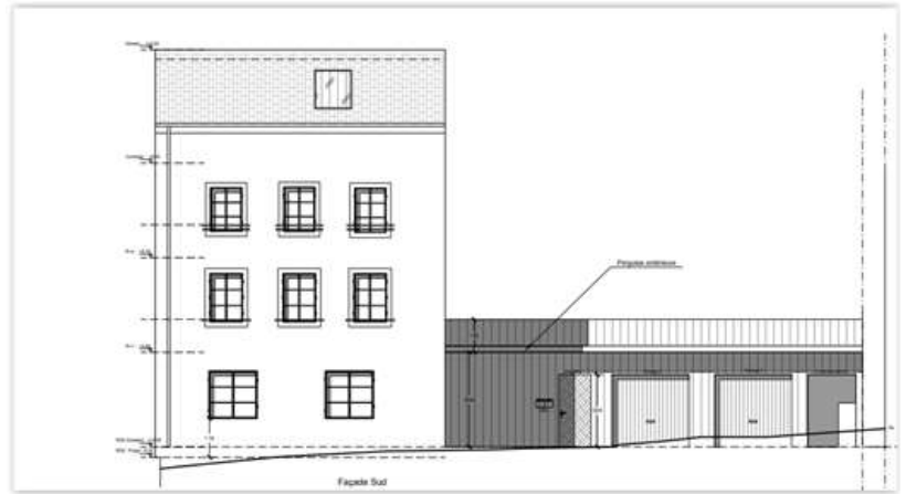
Bâtiments Defix/Oriol : Rez-de-chaussée, un logement de type T3 d'une surface de 78 m 2 . Vue sur RD 590.
