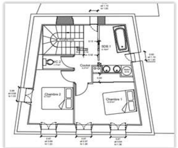
Etages : accès par escalier extérieur sous pergola, appartement de type T4 d'une surface de 106 m 2 + terrasse de 42 m 2 .
