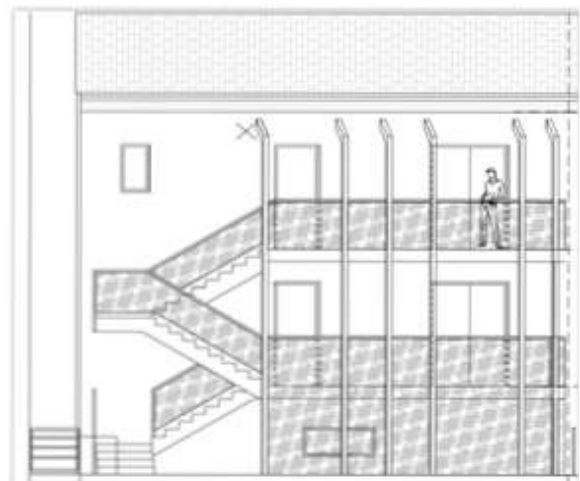
Vue de l'arrière : accès aux appartements
